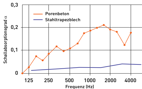
Schallabsorptionsgrade im Vergleich
