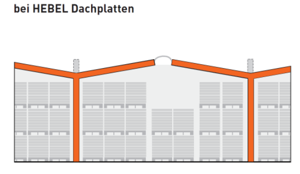
Brandwandkonstruktion ohne Überstand bei HEBEL Dachplatten
